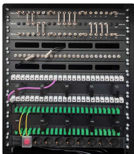
▲ ATE ou PDS em Bastidor 19"
