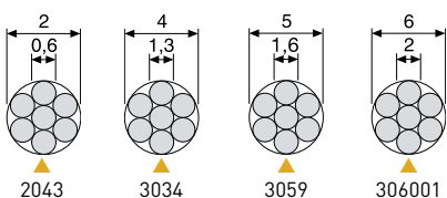
Cabos de aço galvanizado (mm)
